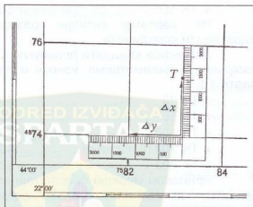
Сл.5.6. Одређивање координата помоћу координатомера
