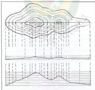
Сл. 5.18. Цртање профила: а) природни, б) неприродни
