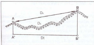
Сл.5.1. Врста растојања
