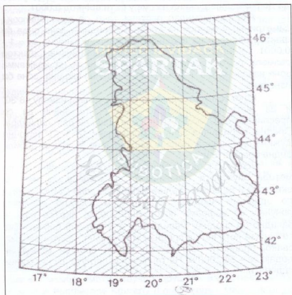
Сл.3.7. Меридијанске зоне
