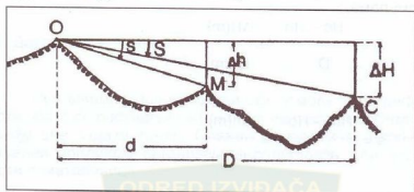
Сл.5.15. Негативни месни углови
