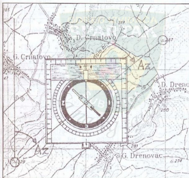
Сл. 5.9. Мерење азимута ручном бусолом
